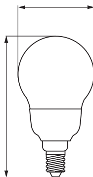
45 mm - E14-04W-G45-WW
