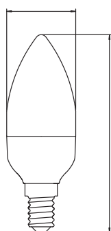
37 mm - E14-04W-C37
